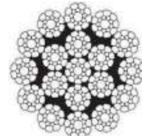
18X19+FC
