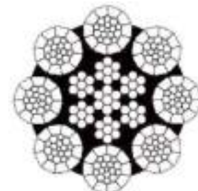
8XWS(26)+IWRC
