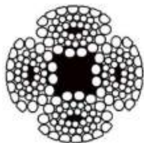
4XSES(39)+FC
