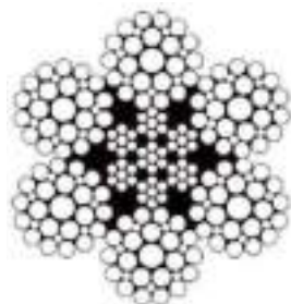
6X29(FI)+IWRC
