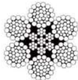
6X36(WS)+IWRC
