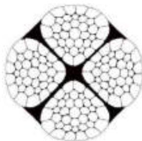
4X36+FC
