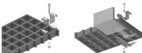
M - type
