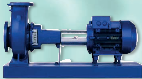
ETANORM centrifugalpumpe
