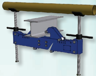
Pipe Rack Jack - Løfteanordning til rør
