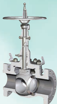
Cameron Orbit kugleventil
