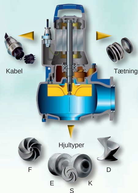
AMAREX N Dykket spildevands- pumpe
