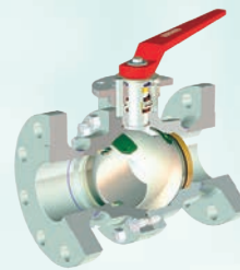
Argus FK 75 kuglehane
