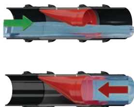
WaStop tilbageløbsventil
