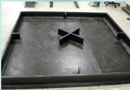
Dobbelt bund til pumpestation - bunden bliver opfyldt med beton
