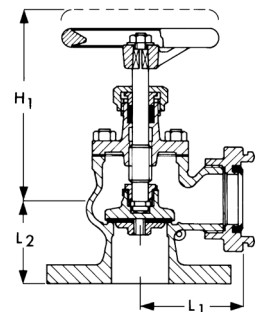
Fig. 912 HOSE ANGLE PN 16
