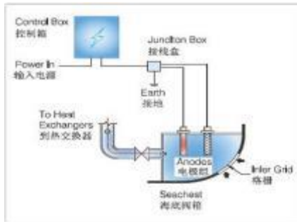
Sea chest Anode Diagram 海水阀箱安装方式
