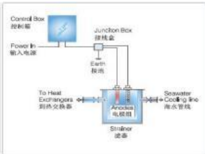
Strainer Anode Diagram 过滤器安装方式
